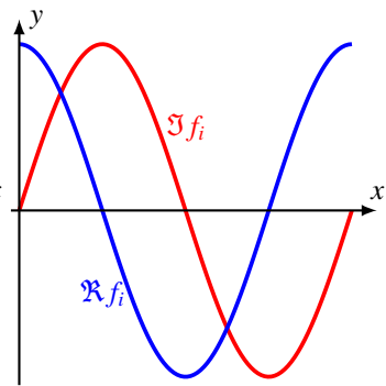
Eigenbasis
