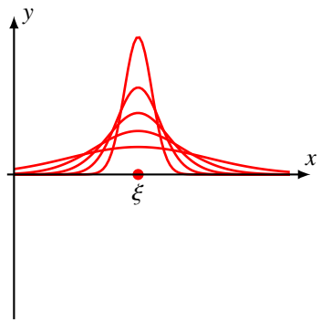
Fundamentallösung
