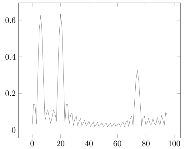
Locator
