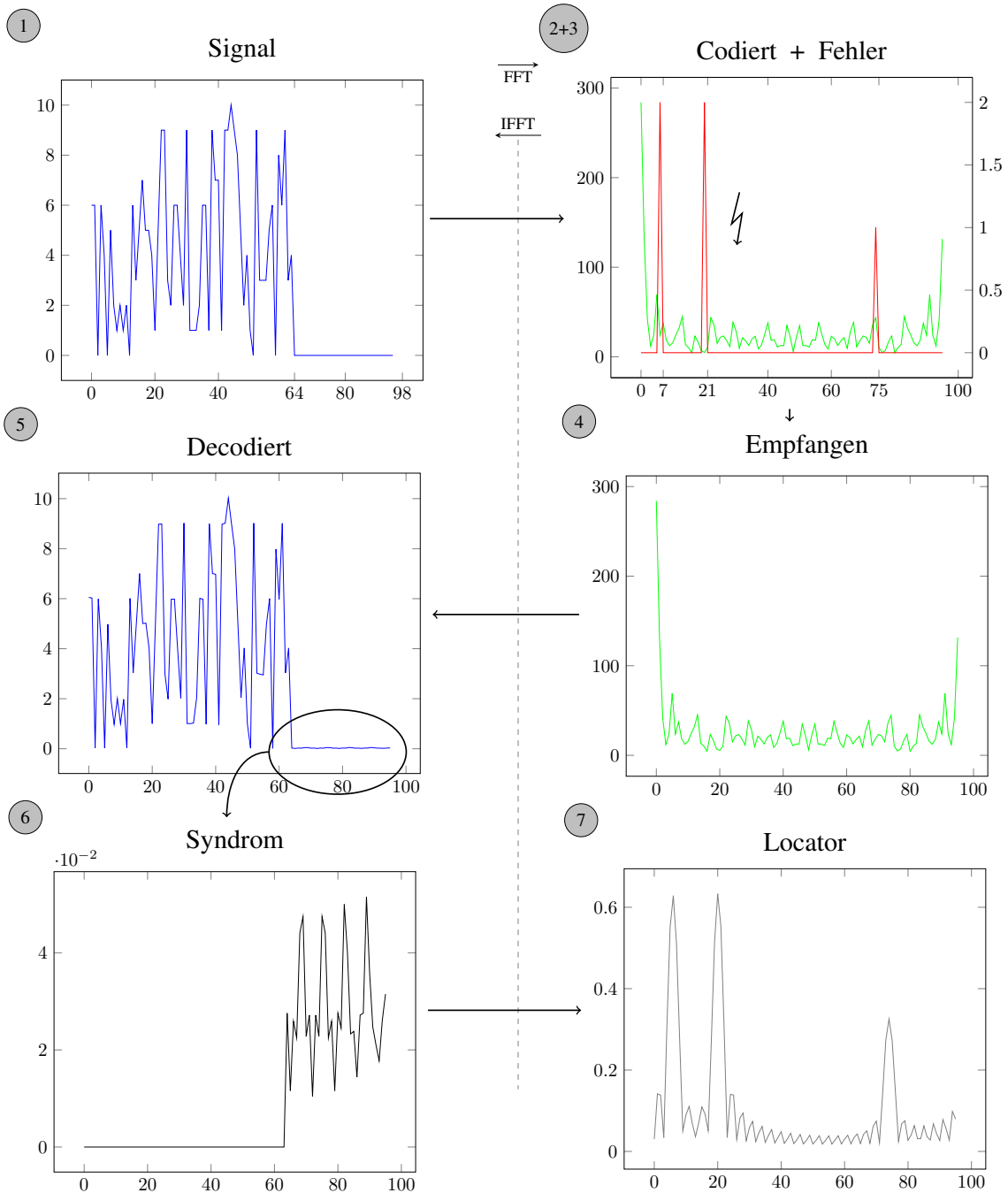
Abbildung 1.2: Übertragungsabfolge 1.4.1
