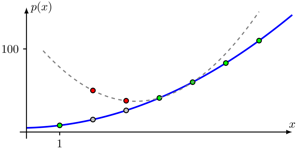
Abbildung 1.1: Polynom p(x) (1.1)
