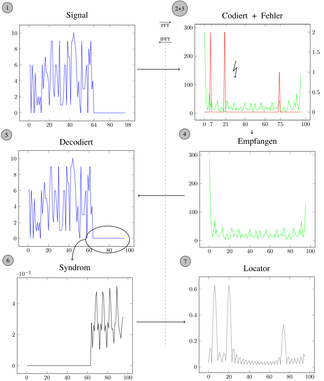
Abbildung 1.2: Übertragungsabfolge ??
