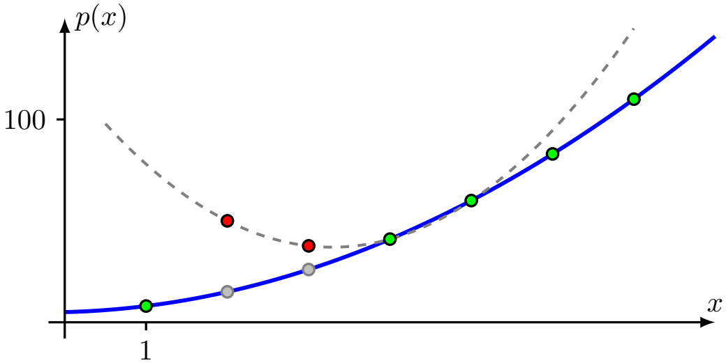
Abbildung 1.1: Polynom p(x) von der Gleichung(1.1)
