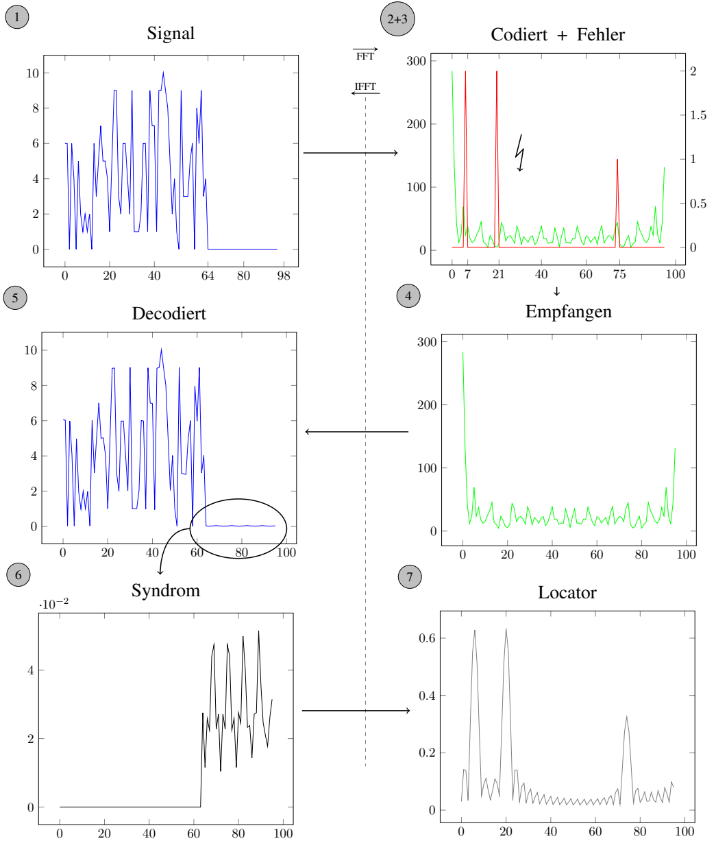
Abbildung 1.2: Übertragungsabfolge 1.4.2
